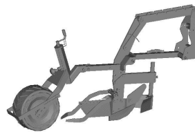
تجهیزات کاشت دانه های درشت (ذرت کار ۱۱۰۹)
